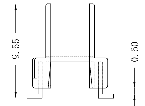
脚型A: 缠线高度0.60 骨架总高9.55
