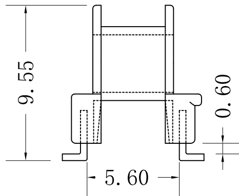
脚型A缠线高度0.60 骨架总高9.55
