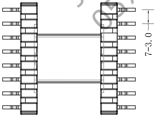
脚型B 全针料号PF-EFD2020M28.85BK0
