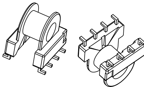
脚型B: 缠线高度0.90 骨架总高9.85
