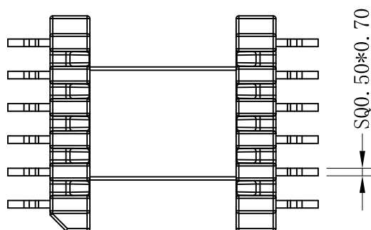
脚型B 挂线空间1.4, 排距做28.85
