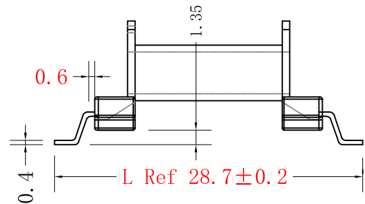
脚型C 全针料号PF-EFD2020M28.7CK0
