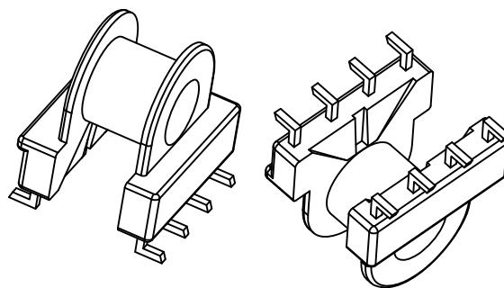
脚型B:缠线高度0.90 骨架总高9.85
