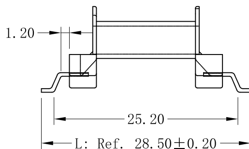
脚型A 挂线空间1.2, 排距可做28.50
