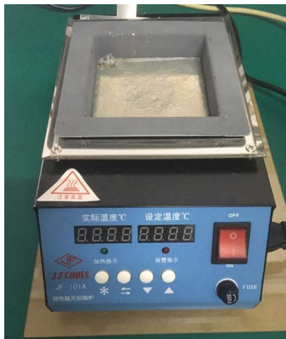
易上锡性及耐烫锡试验
