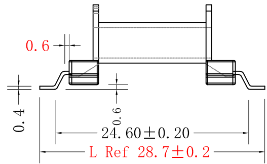
脚型A 全针料号PF-EFD2020M28.7AK0
