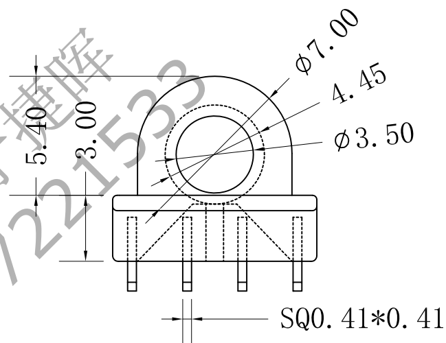
脚型A缠线高度0.60 骨架总高9.55
